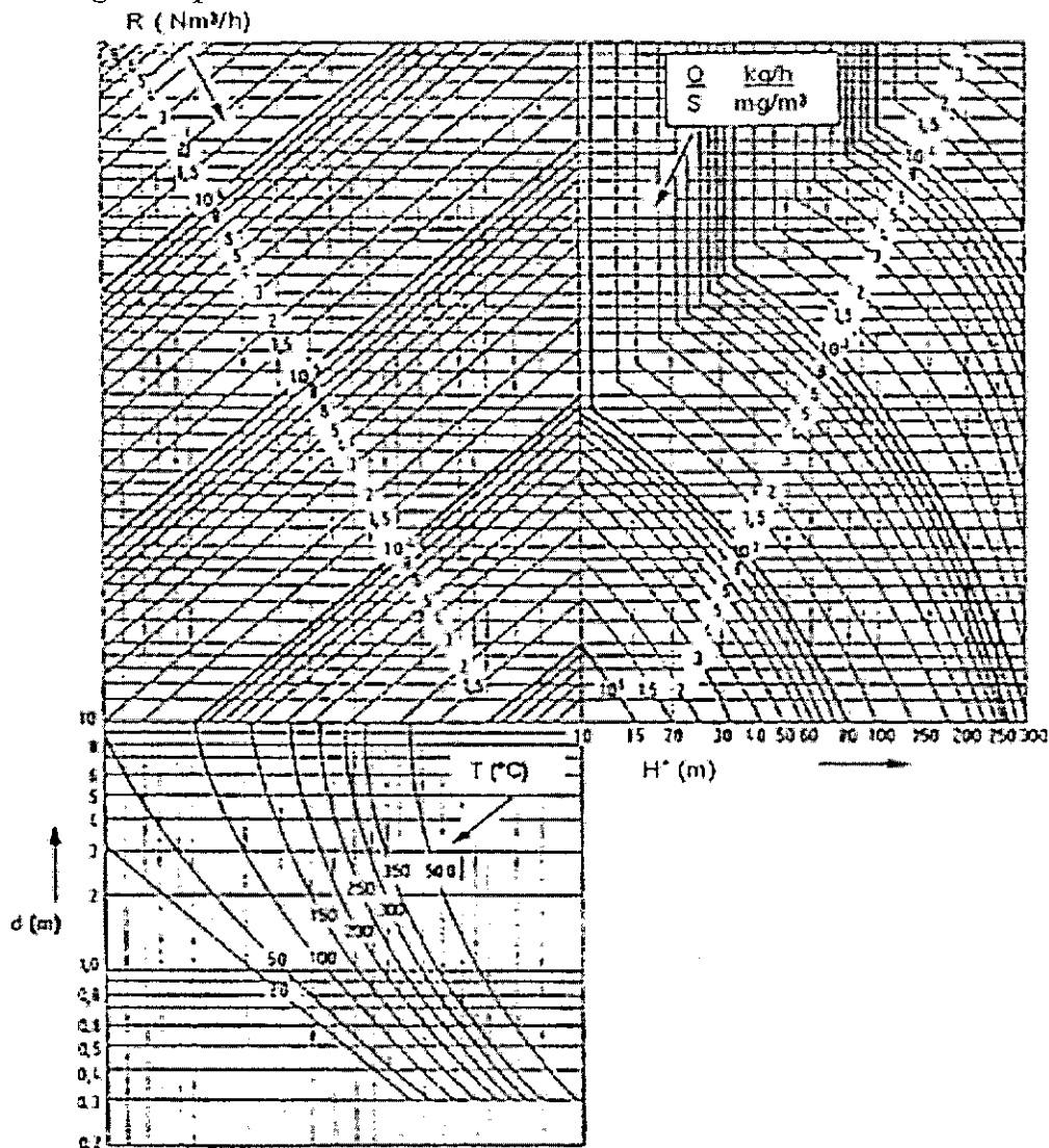
Gráfica 1. Nomograma para el cálculo de la altura mínima de chimenea.
