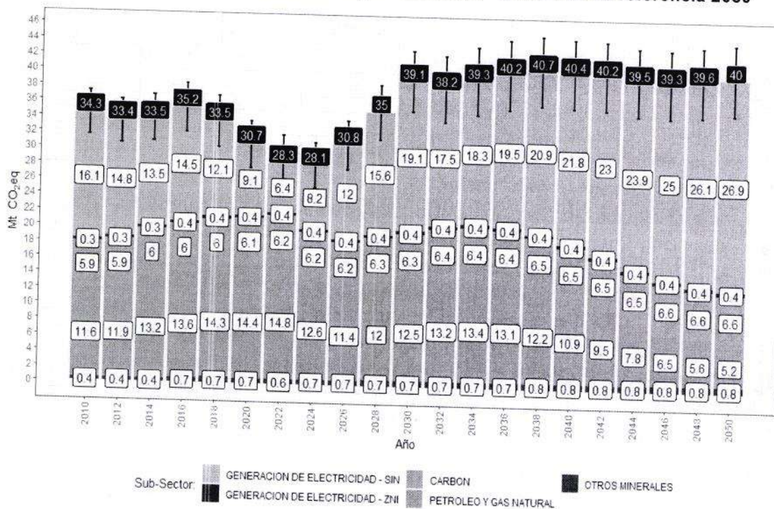
Figura 2. Proyección de emisiones GEI por subsector - Escenario de referencia 2050
