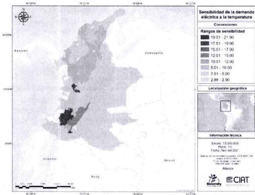
Figura 6. Resultados de los modelos de regresión para la variable consumo promedio como referencia por departamentos
