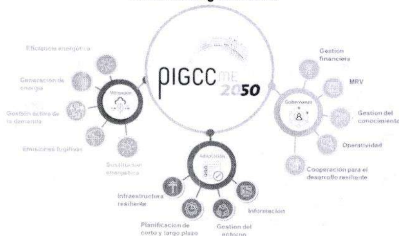
Figura 8. Esquema del Plan Integral de Gestión del Cambio Climático del Sector minero energético 2050
