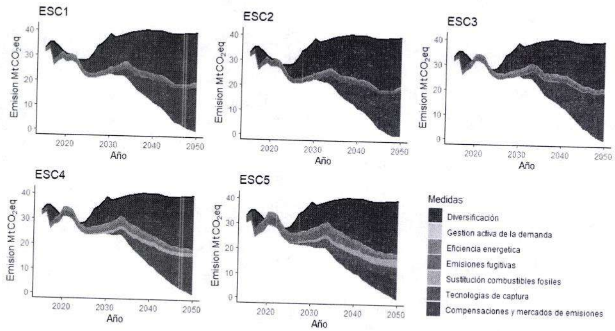
Figura 5. Sendas probables de carbono neutralidad del sector minero energético
