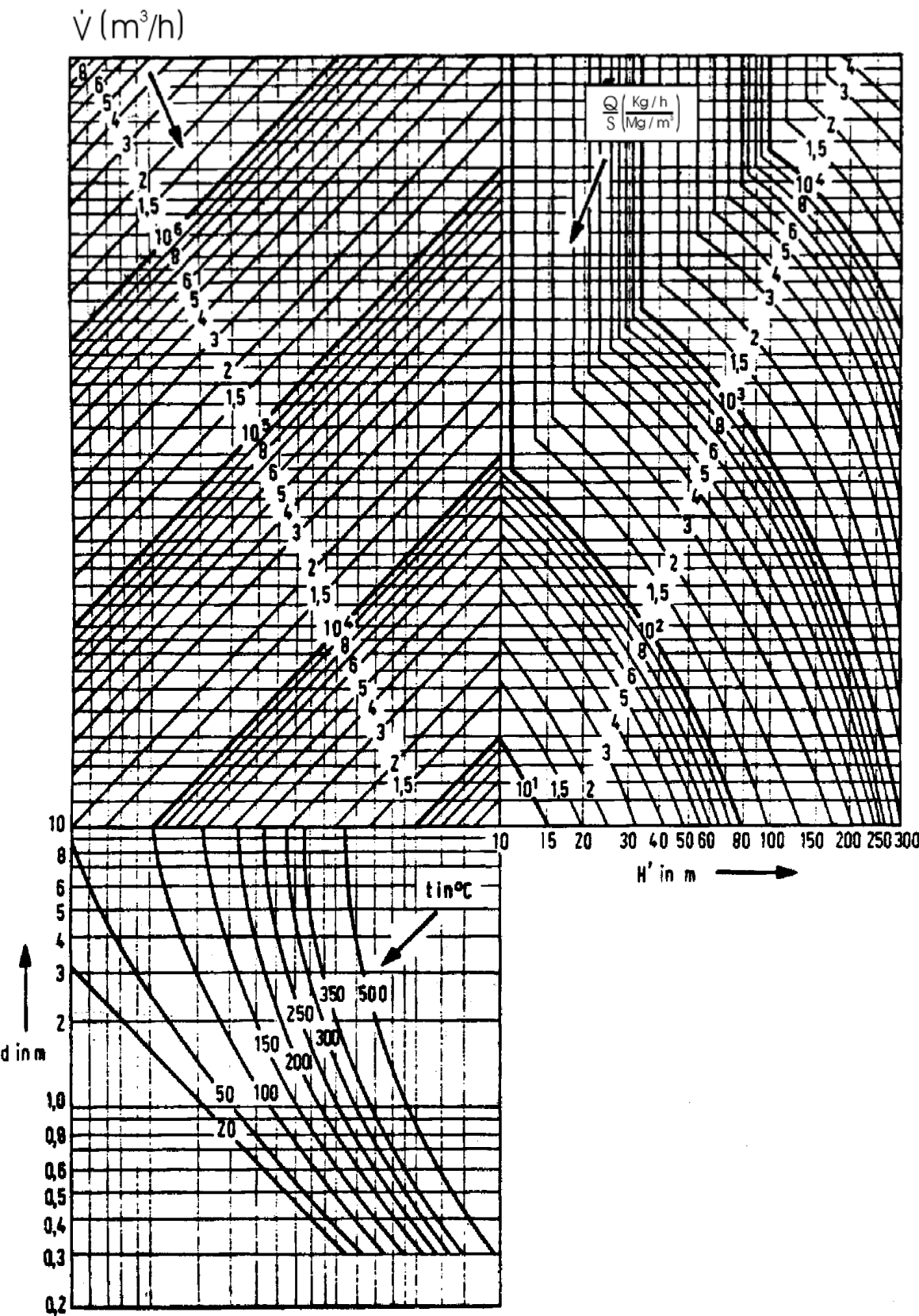
Figura 1. Nomograma para cálculo de altura mínima en chimeneas. FUENTE: Guía Ambiental Alemana de Control de Polución del Aire (TA LUFT-Technische Anleitung zur Reinhaltung der Luft), C.H. Beck Verlag, Munchen 1987, Alemania
